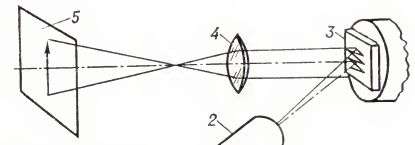
Рис. 8. Схема проекционного лазерного телевизора: 1 — электронная пушка; 2 — фокусирующая и отклоняющая система; 3 — полупроводниковый кристалл — резонатор; 4 — объектив; 5 — экран.
